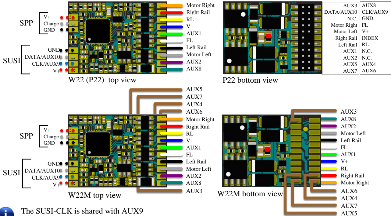
Figure 5: Lokommander II Mini P22, W22 and W22M
